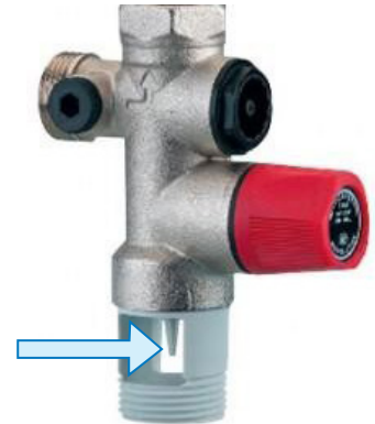
Veiligheidsgroep met overdrukventiel
